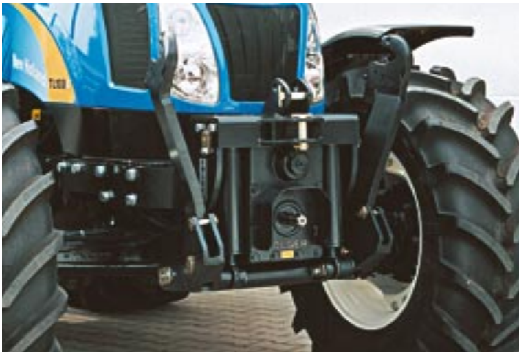
Anlenkpunkt vom Unterlenkerträger sehr nahe an der Vorderachse. Hohe Bodenfreiheit.
